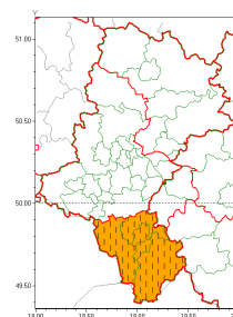
Zawieje/zamiecie śnieżne 2022-01-30 20:47
